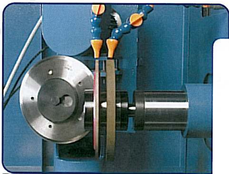
Vor- und Fertigschliff in einer Aufspannung.
